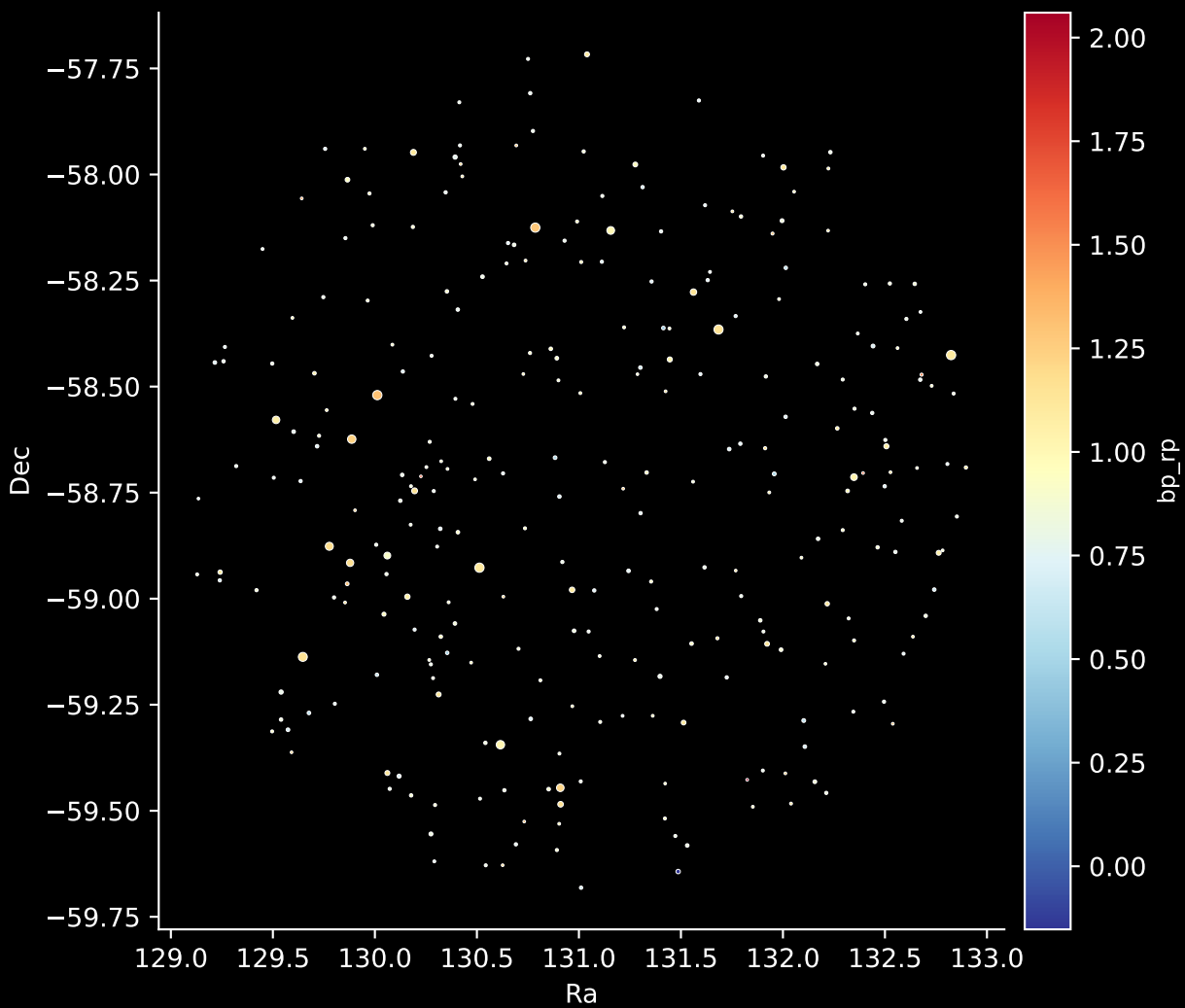
GALAH DR4 Field: [6887] Stars: 279
