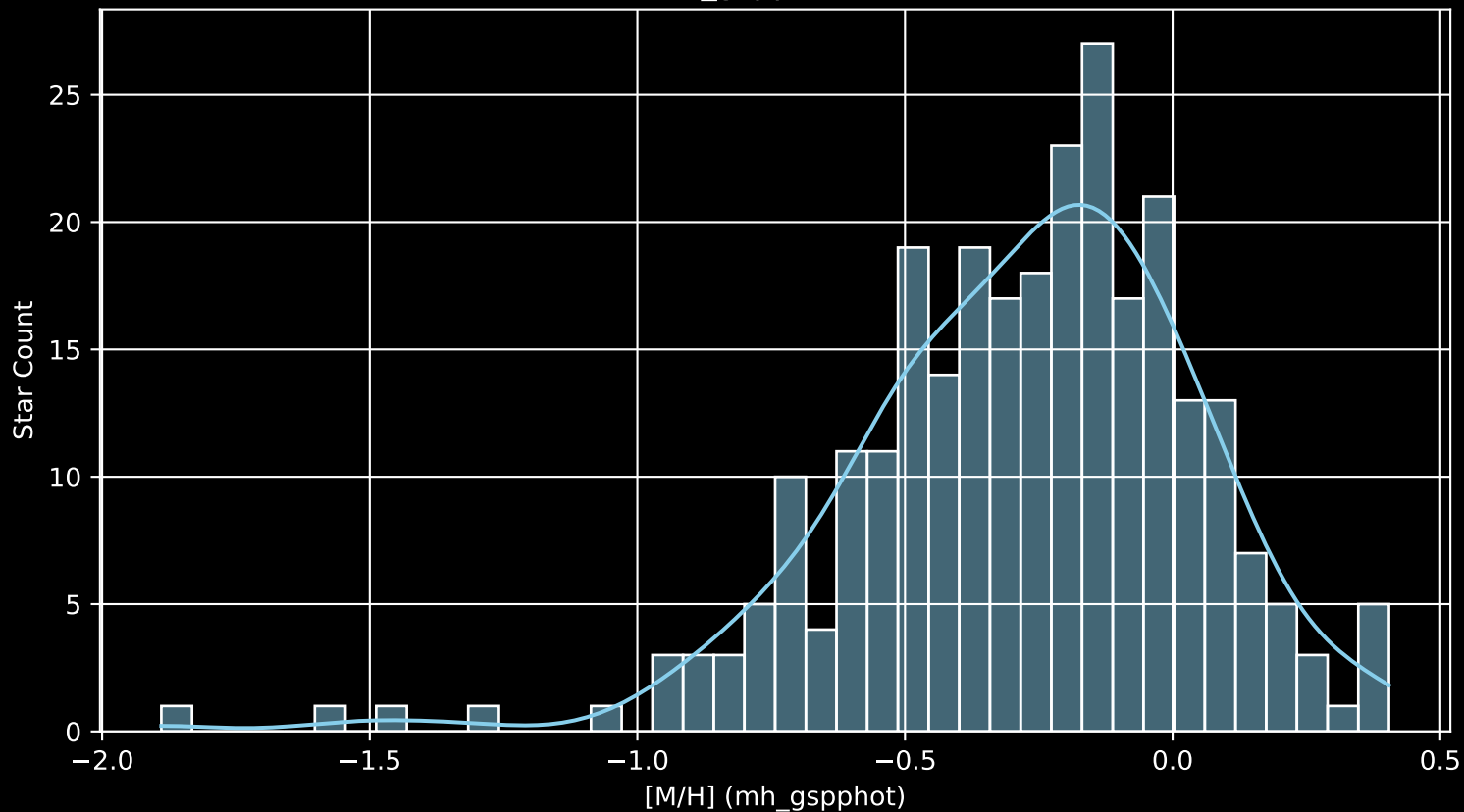
GALAH DR4 Field: [6887] [M/H] (mh_gspphot) (n= 277)
