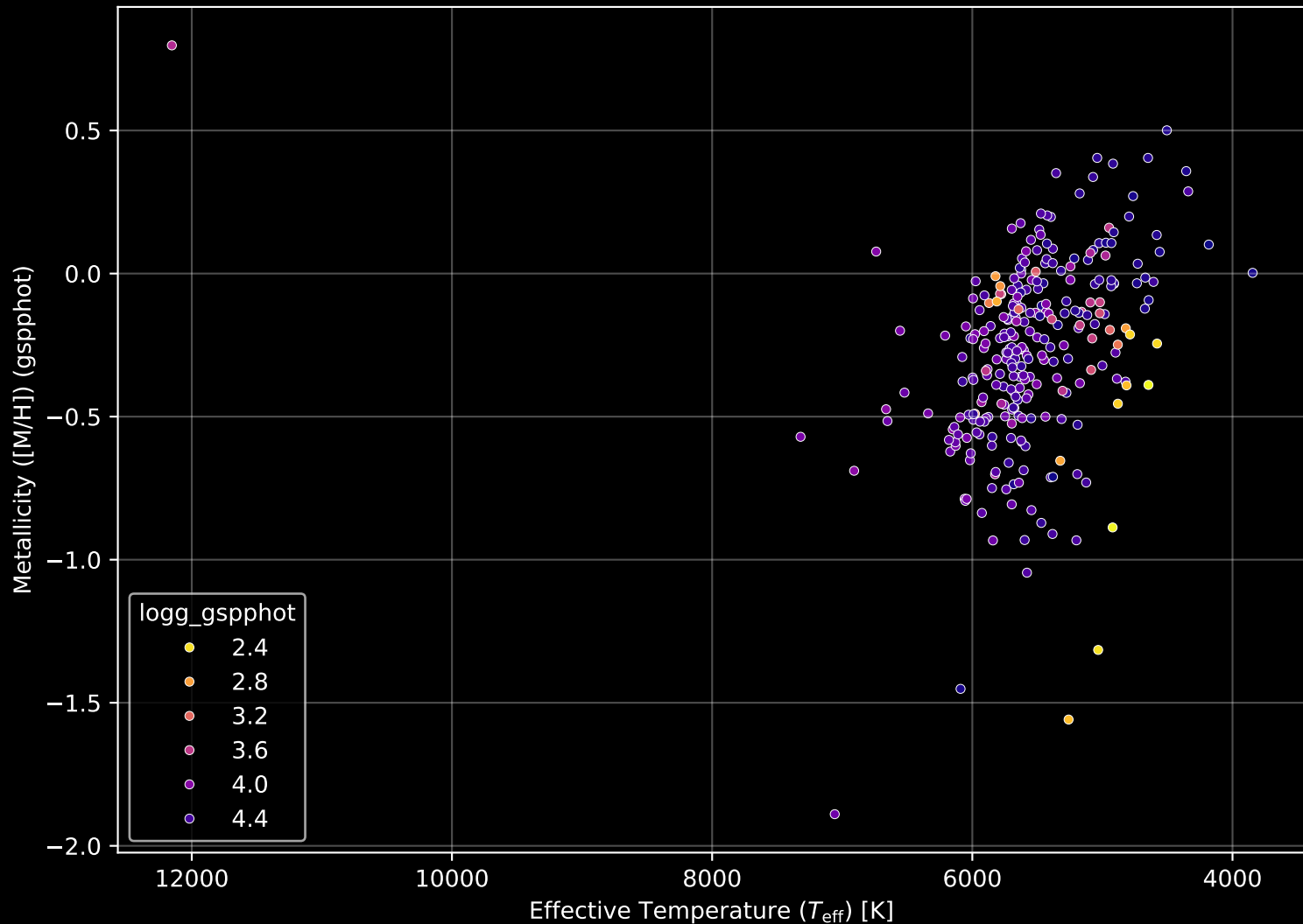
GALAH DR4 Field: [6887] Stellar Population Parameters (n= 279)
