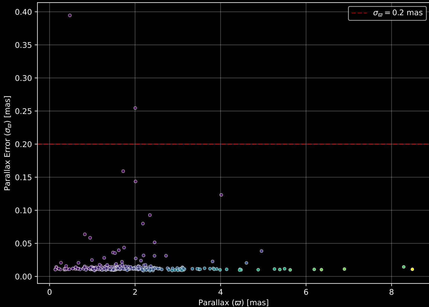
GALAH DR4 Field: [6887] Parallax Quality (n= 279)
