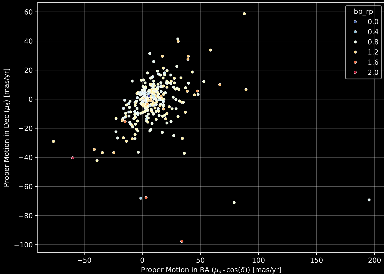
GALAH DR4 Field: [6887] Proper Motion Diagram (n= 279)
